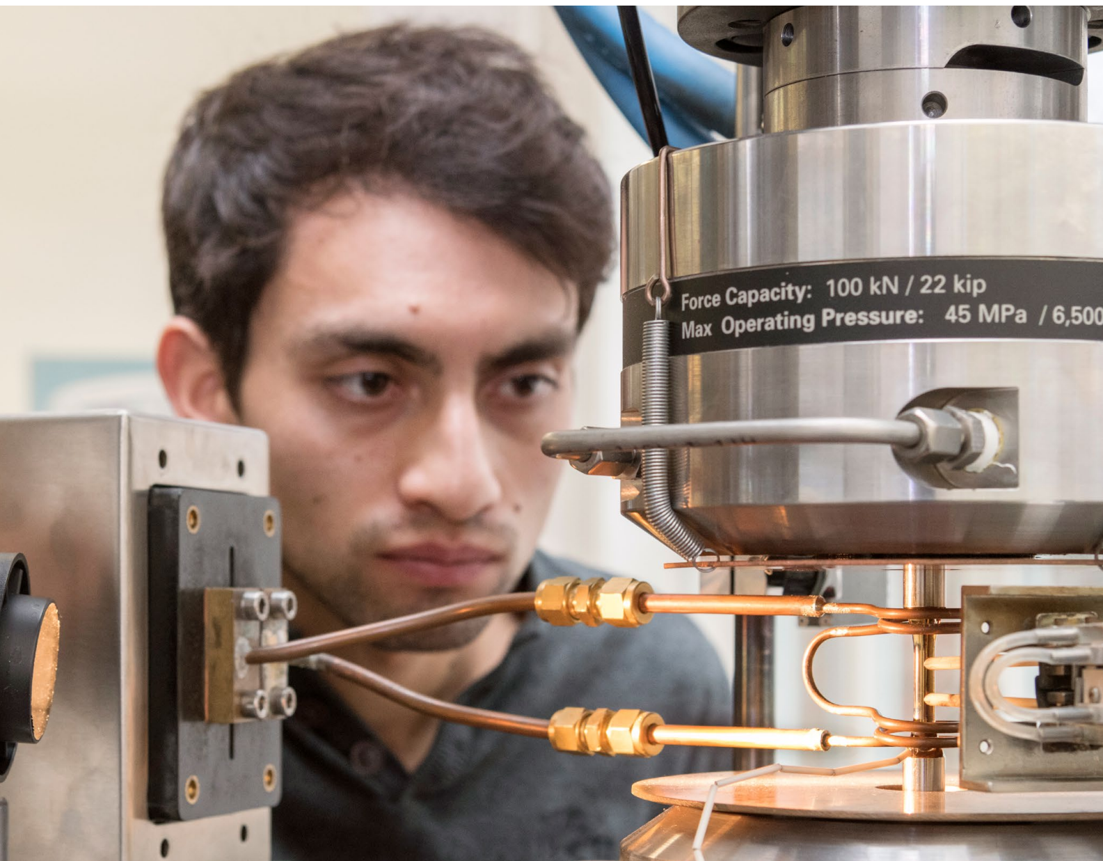
Mechanische Hochtemperaturprüfung von additiv gefertigten Proben
