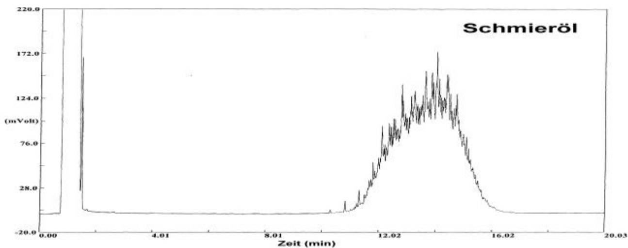
Abb.2: GC/FID-Chromatogramm von BAM KS 5003 Schmieröl
