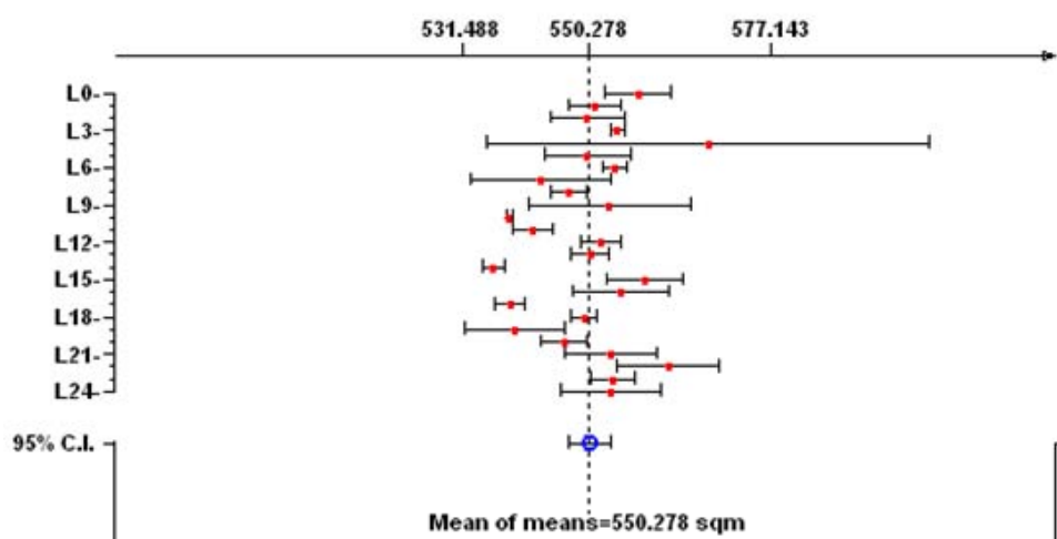
Abb. 7 Auftragung der Messplatzmittelwerte für BAM-P108 als SoftCRM-Grafik [9]. Die Unsicherheitsbalken zeigen hier die 95%-Vertrauensintervalle (95% C.I.) der jeweiligen Mittelwerte (rot). Blau dargestellt ist der Mittelwert der Messplatzmittelwerte (Mean of the means) mit seinem C.I. Die Zahlenangaben auf der Abszisse kennzeichnen den Mittelwert der Messplatzmittelwerte sowie den kleinsten und größten Einzelwert aller Messplätze als Spannweite.
