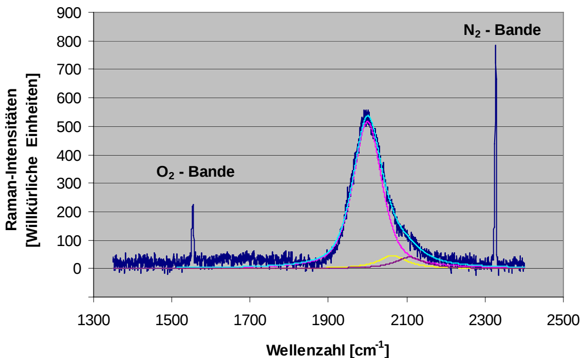
Abbildung 4.3: \text{SiH}_x – Bande der amorphen Si – Schicht mit Bandenfit für x = 1 (magenta), x = 2 (gelb), x = 3 (lila) und die Summe (hellblau) ( \text{O}_2 - und \text{N}_2 - Bande siehe Text)
