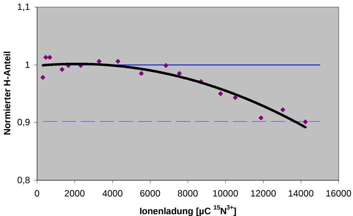
Abbildung 4.5: Abhängigkeit des normierten Messwertes von der akkumulierten Ionenladung für Probe a.26: gefitteter Trend (durchgezogene Linie), zertifizierter Wert (durchgezogene Gerade) und dazugehörige Messunsicherheit (gestrichelte Linie)
