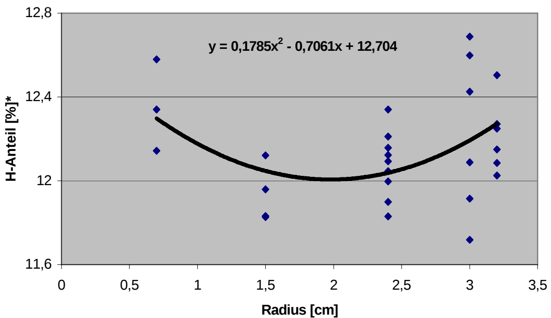
Abbildung 5.11: aSi:H auf Substrat c - Regressionsanalyse der Homogenität des Wasserstoffanteils radial
