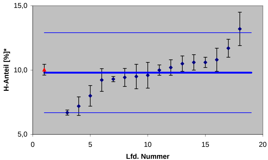
Abbildung 5.5: Zusammenfassung der Messergebnisse des Ringversuchs für den Wasserstoffanteil für aSi:H auf Substrat b * früher auch als at.% bezeichnet
