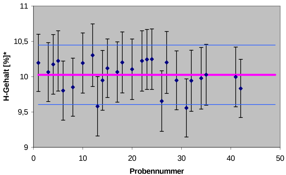
Abbildung 5.2: Wasserstoffanteil in den Proben aus dem beschichteten Substrat b * früher auch als at.% bezeichnet
