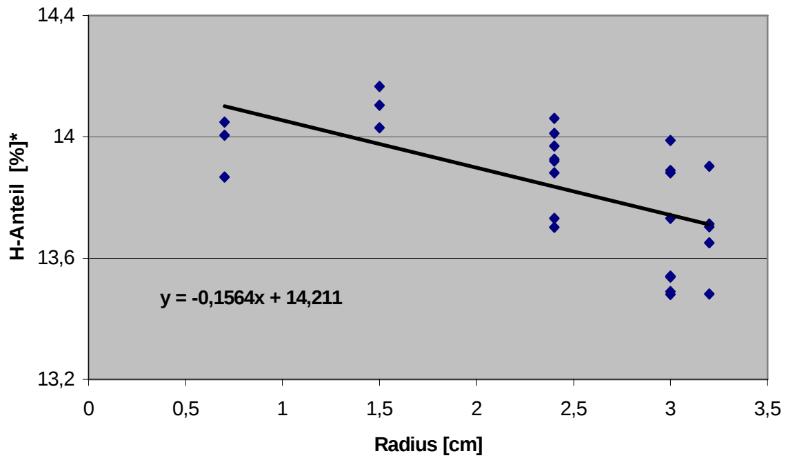
Abbildung 5.10: aSi:H auf Substrat a - Regressionsanalyse der Homogenität des Wasserstoffanteils oben-unten
