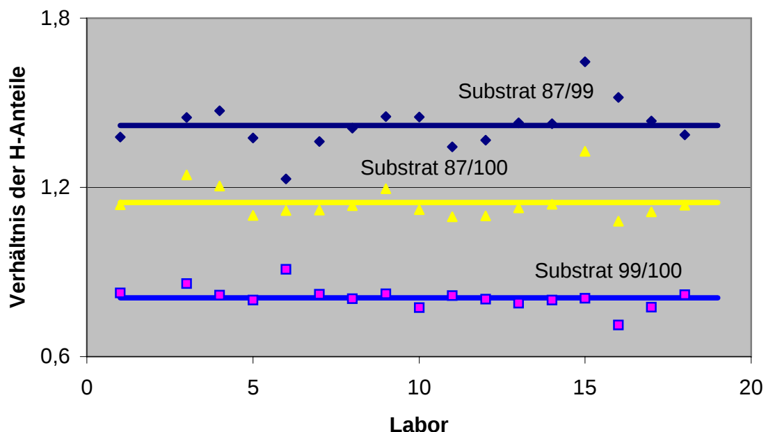
Abbildung 5.7: Verhältnisse der gemessenen Wasserstoffanteile in den Schichten auf den Substraten a, b und c
