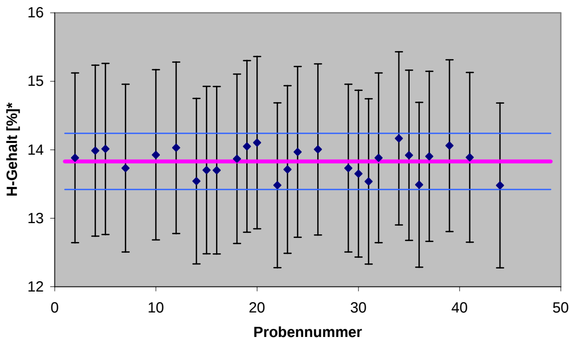
Abbildung 5.1: Wasserstoffanteil in den Proben aus dem beschichteten Substrat a * früher auch als at.% bezeichnet
