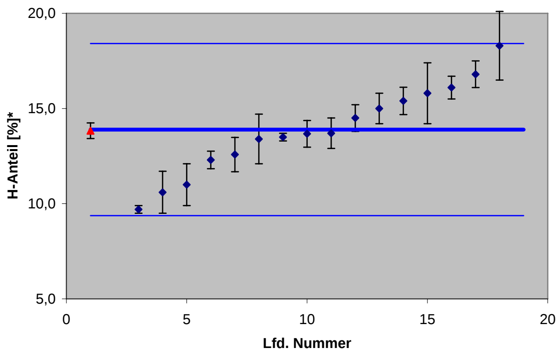
Abbildung 5.4: Zusammenfassung der Messergebnisse des Ringversuchs für den Wasserstoffanteil für aSi:H auf Substrat a
