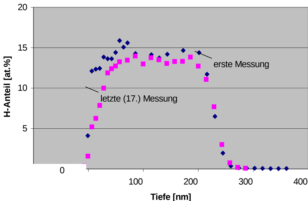
Abbildung 4.6: Veränderungen im Profil des Wasserstoffanteils in Abhängigkeit von der Bestrahlung (Ionenfluenz)
