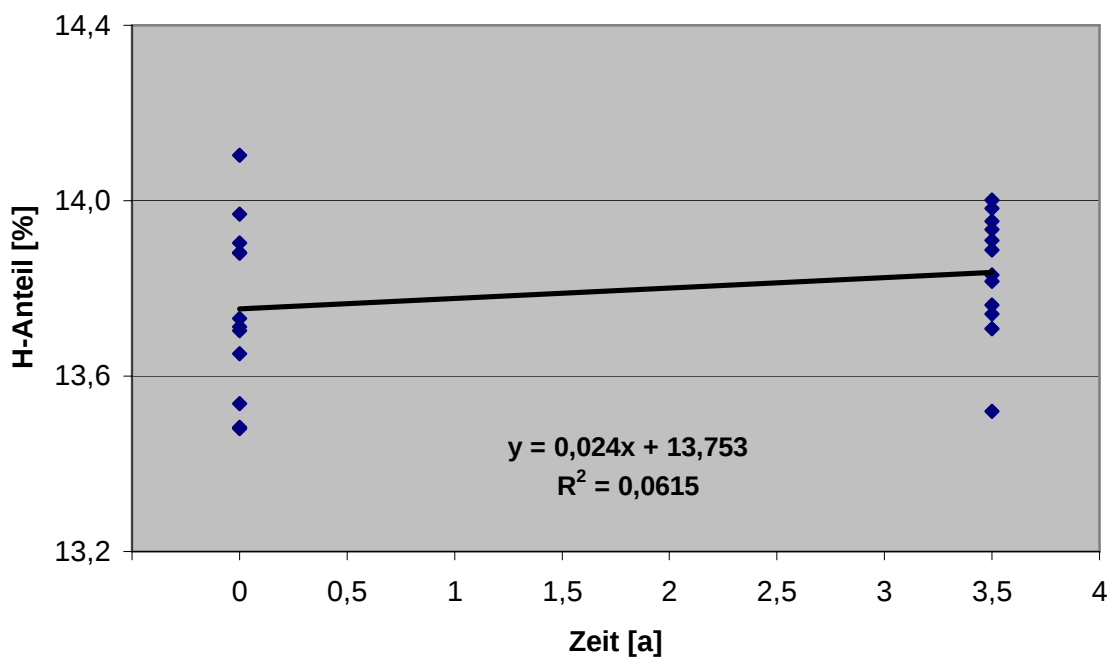
Abb. 4.4: Messdaten und Regressionsgerade zur Untersuchung der Stabilität des Materials
