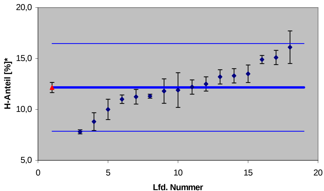
Abbildung 5.6: Zusammenfassung der Messergebnisse des Ringversuchs für den Wasserstoffanteil für aSi:H auf Substrat c * früher auch als at.% bezeichnet
