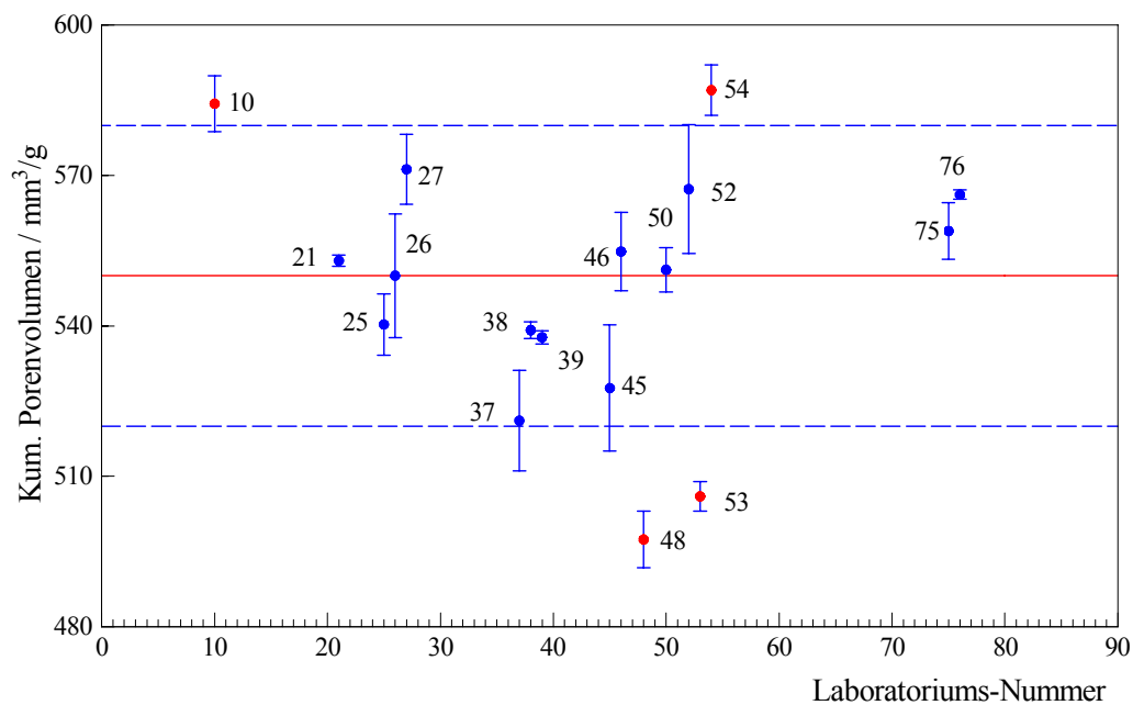
Abb. 15 Eignungstest 1, 400 MPa, Substanz Silica-Alumina, Kenngröße spezifisches Porenvolumen Referenzwert: 550 \pm 30 \text{ mm}^3/\text{g}
