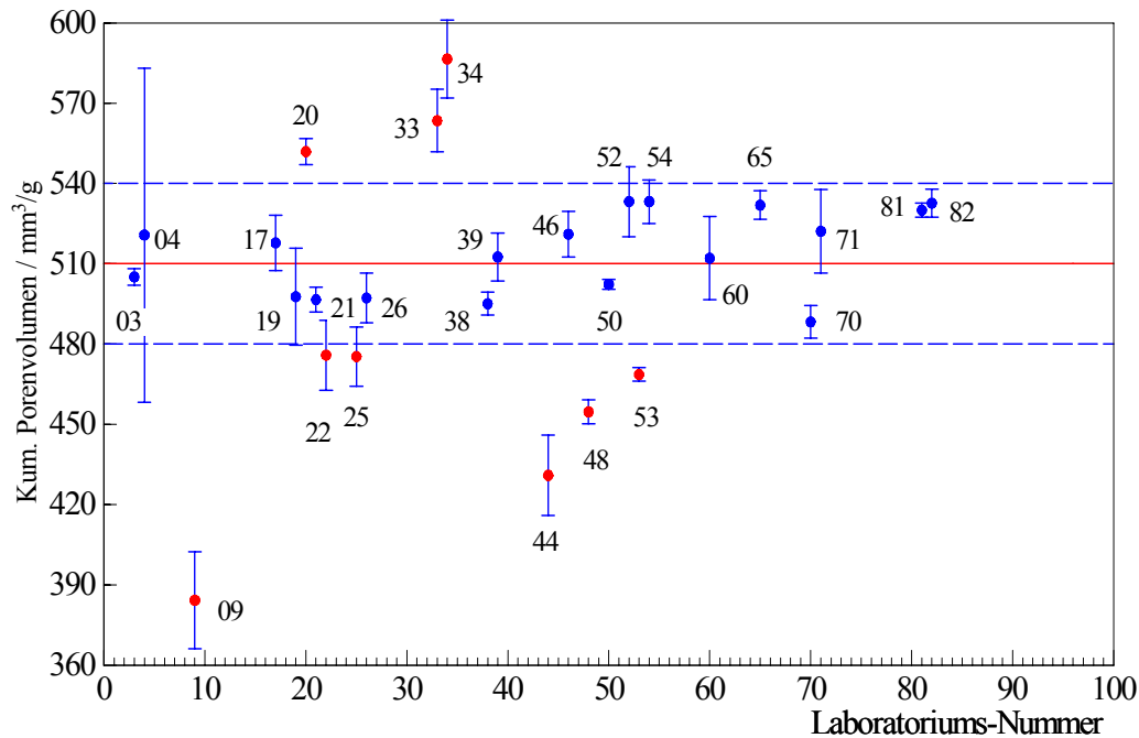
Abb. 14 Eignungstest 1, 200 MPa, Substanz Silica-Alumina, Kenngröße spezifisches Porenvolumen, Referenzwert: 510 \pm 30 \text{ mm}^3/\text{g}
