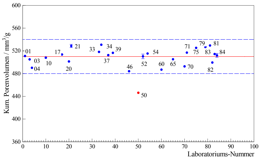
Abb. 17 Eignungstest 2, 200 MPa, Substanz Silica-Alumina, Kenngröße spezifisches Porenvolumen, Referenzwert: 510 \pm 30 \text{ mm}^3/\text{g}
