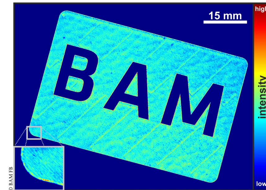
Einzelbild der optischen Tomografie, aufgenommen bei einer Wellenlänge von 880 nm. Dies ist eine Langzeitbelichtung über den Aufbau einer gesamten Lage eines Demonstrationsprobekörpers, in dem der Schriftzug „BAM“ als pulvergefüllter Hohlraum verbleibt. Inset: Detaildarstellung.
