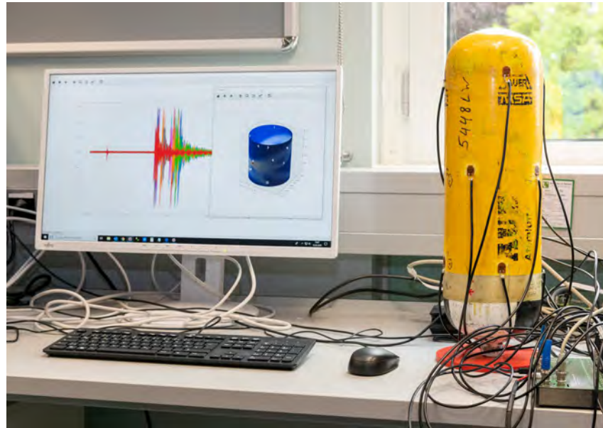
Versuchsaufbau mit Demonstrator Lab demonstrator
